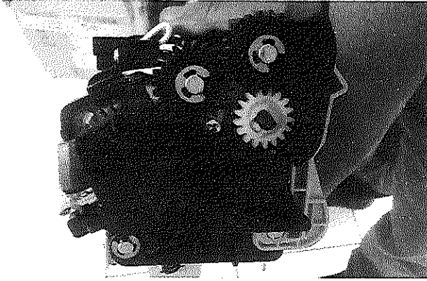
FOTOSENSOR NUEVO
